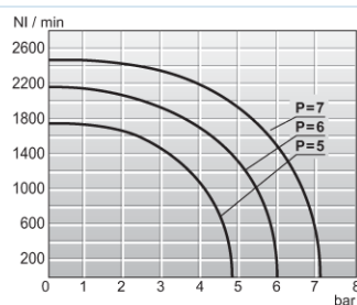
Átfolyási diagramm 1/4"
