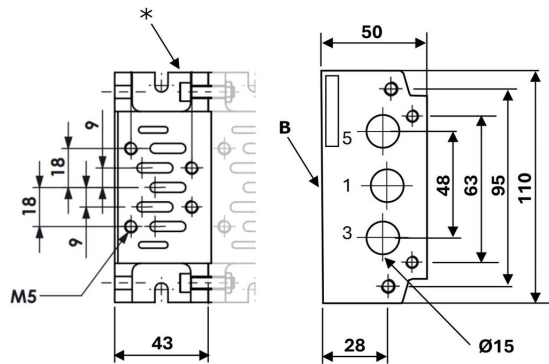
Középrész SBI1-CE típusú
