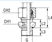
med B4-skærering
