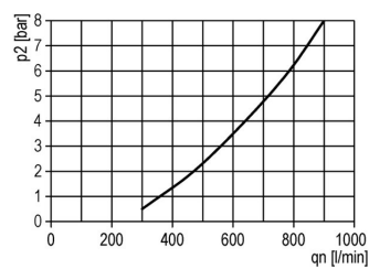
Öljysumuttimen toimintaraja
