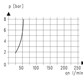
Öljysumuttimen toimintaraja
