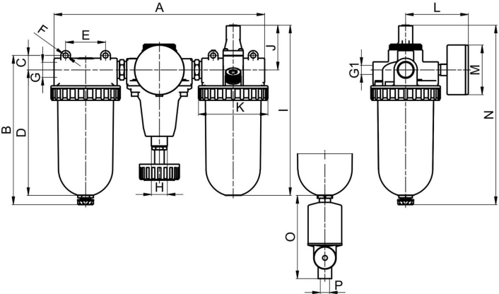
purgeur automatique
