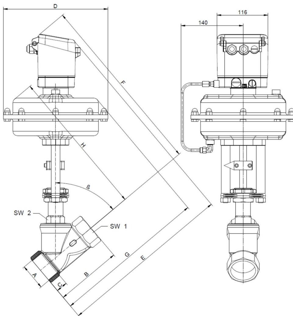
Membrantrieb D250 mit digitalen Stellungsregler 8049
